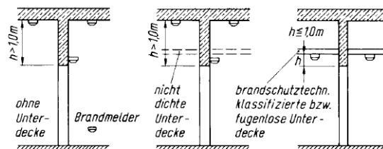
Bild 1: Maßgebende Höhe der Deckenunterfläche
