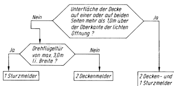
Bild 3: Entscheidungsdiagramm zu 4.1.1
